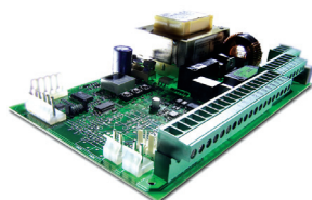
Stuurprint 624 BLD (ingebouwd) Specificaties zie p. 194
